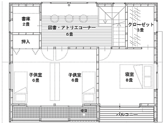
2階平面図
